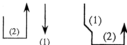
図5-1 2本のバイトで加工 図5-2 1本のバイトで加工
