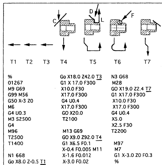
図8 ベアリングの加工レイアウトとプログラム
