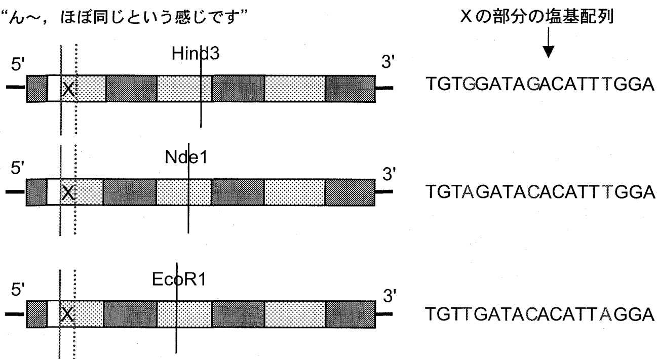
図 2 3 つの DNA 断片における X 部分の塩基配列 (TC2 genome DNA) の構造
