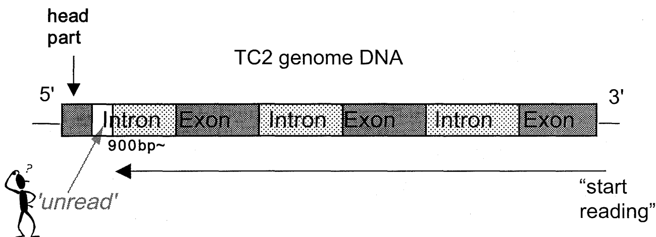
図1 NKの実験対象：植物のカフェイン合成ゲノム遺伝子 (TC2 genome DNA) の構造
